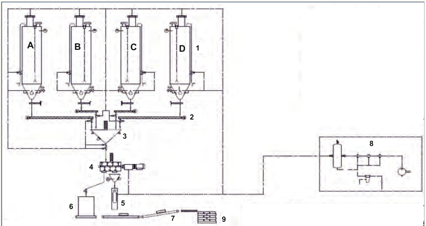
VÝROBA SUCHÝCH HMOT - příklad Základní výrobní modul BPM
